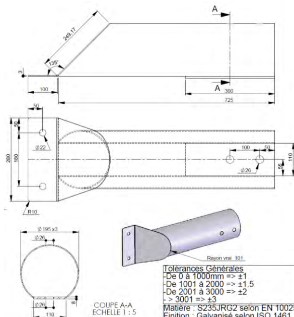
Queue de carpe à spiter (spécial GBA ou mur béton)
